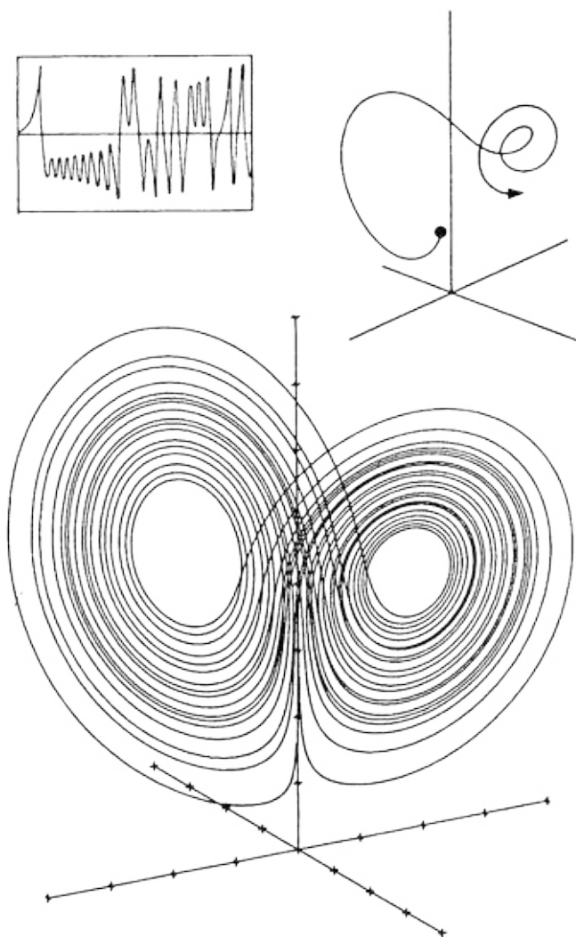
Рис. 1.4. Аттрактор Лоренца. Это магическое изображение (внизу), напоминающее маску
