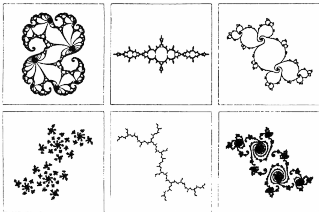
Рис. 8.1. Примеры изображений, полученных с помощью множеств Джулиа.
