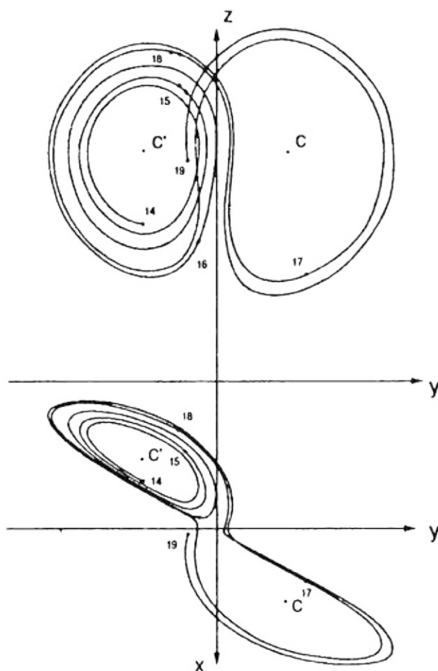
Рис. 5.3. Первый странный аттрактор. В 1963 г. Эдвард Лоренц смог вычислить только первые несколько элементов аттрактора для своей простой системы уравнений. Однако он
