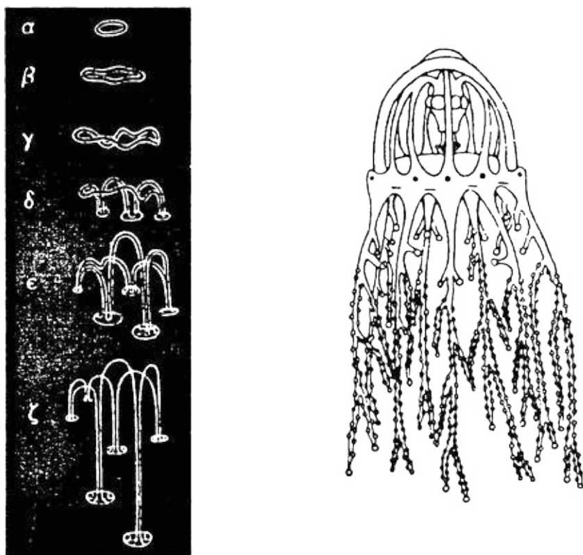
Рис. 7.1. Падающие капли. Д'Арси Вентворт Томпсон продемонстрировал висячие нити и столбики, которые можно увидеть и у попавшей в воду капельки чернил (слева), и у медузы (справа). «Чрезвычайно любопытный результат... Он показывает, как чувствительны... эти капли к физическим условиям. Используя все время один и тот же желатин и варьируя лишь плотность жидкости в пределах тысячных долей, мы получаем целый ряд конфигураций — от обычной висящей капли до капли с рубчатой поверхностью...»
